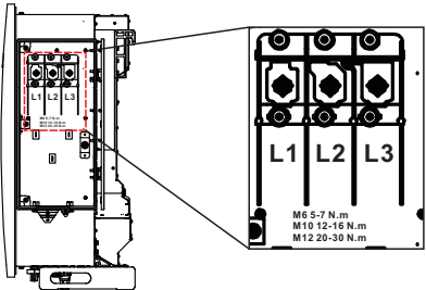
图3.22 交流端子排
