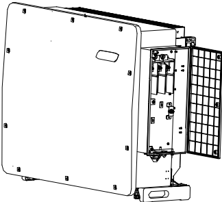
图3.21 拆下接线盒盖
