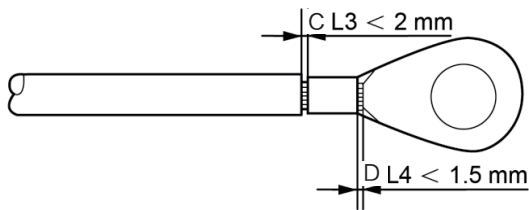
图3.11 线缆压接
