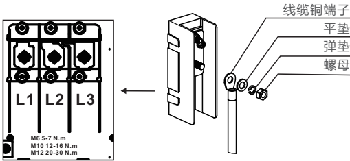
图3.20 铜铝过渡转端子
