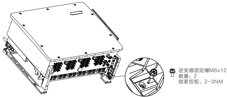
图3.9 固定逆变器
